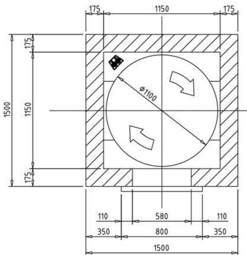
VISTA SEZIONATA IN PIANTA
